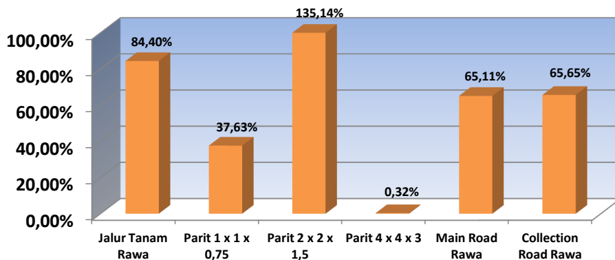
Pekerjaan Excavator
